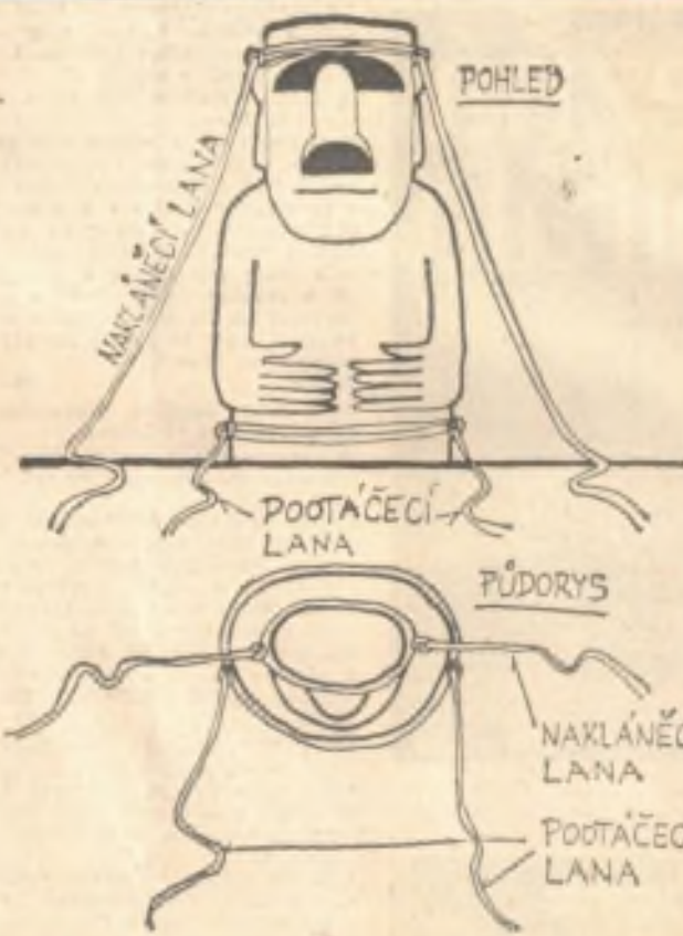
Náčrt principu upevnění lan pro pohyb moai
