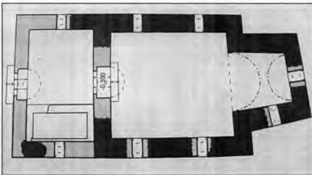
Půdorys kostela sv. Markéty Antiochijské s rekonstrukcí nartexu – předsíně pro katechumeny
