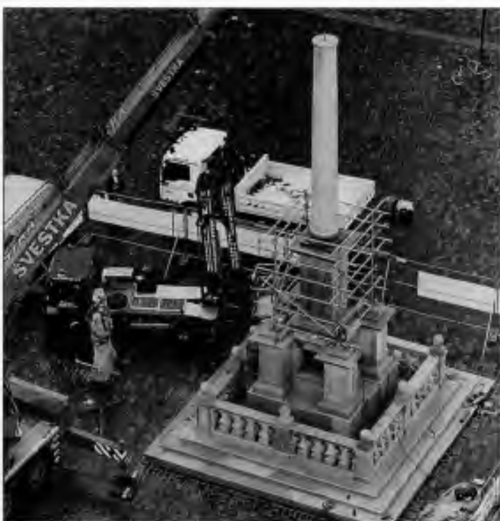
Dřík sloupu vážící 22 tun po umístění na podstavec
