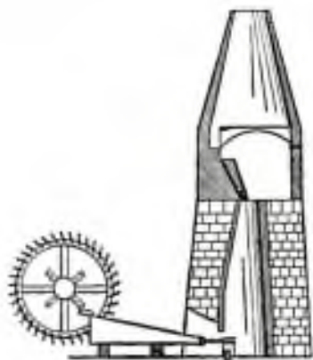
Redukční pec dýmačka s měchem, který byl poháněn vodním kolem
