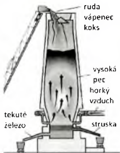
Tavení železné rudy ve vysoké peci
