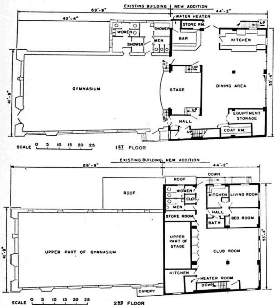
Plán na přístavbu sokolovny v Los Angeles. — Vypracoval br. Karel M. Prchal.
