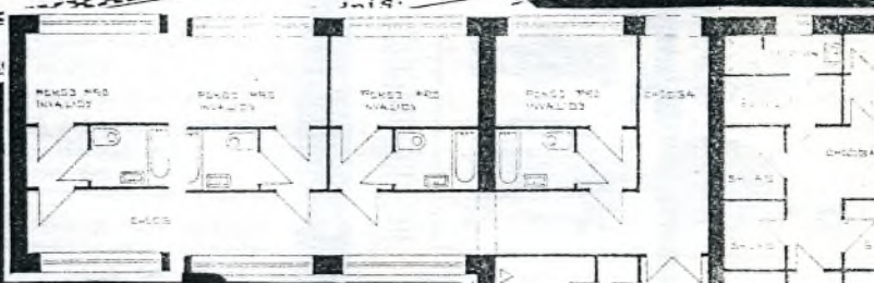
Půdorys přízemní části "DEPA".
