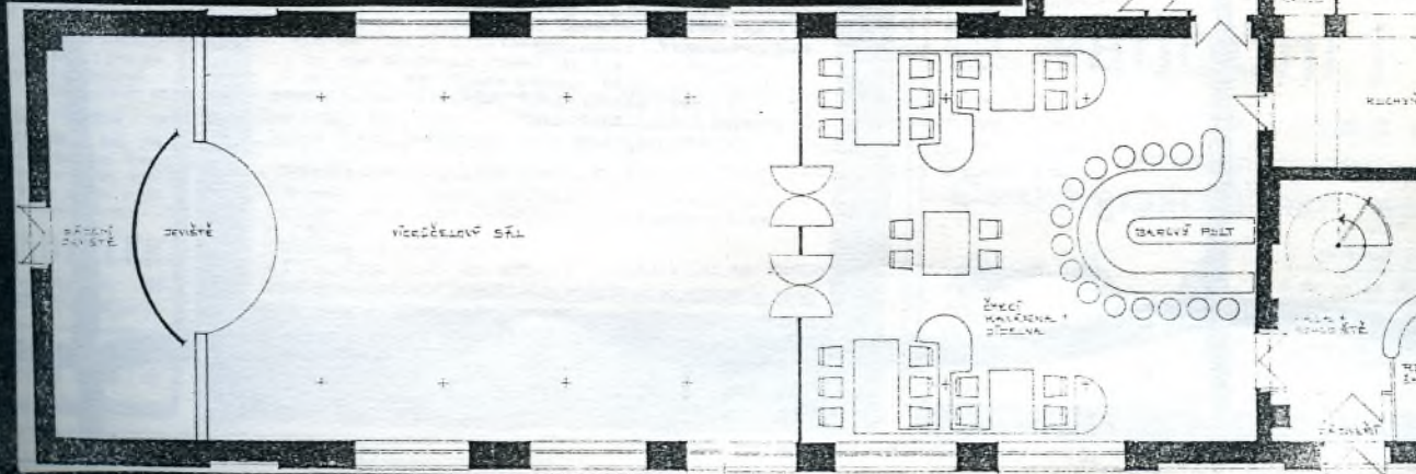
Půdorys přízemní části "DEPA".
